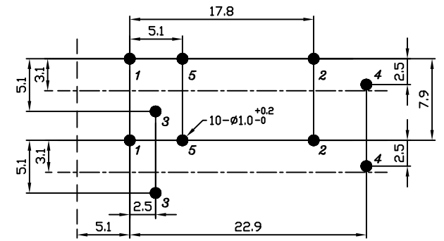
P.C.B LAYOUT(±0.1) (BOTTOM VIEW)
