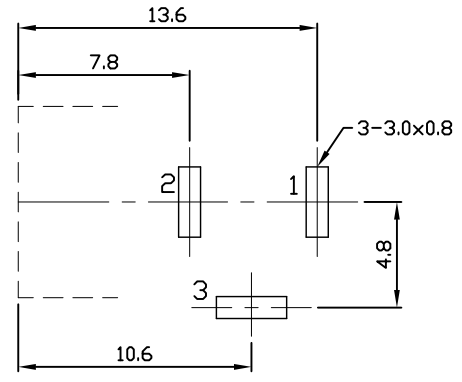
P.C.B LAYOUT(±0.1) (TOP VIEW)
