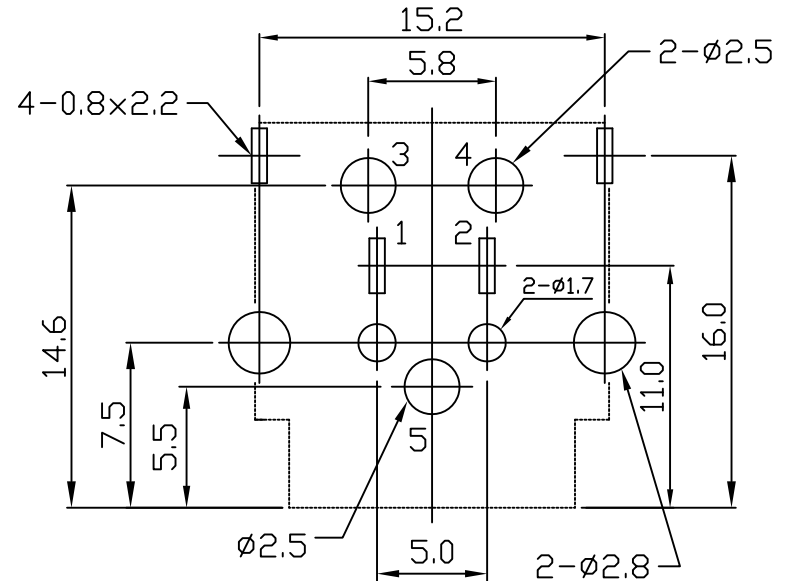
P.C.B LAYOUT(±0.1) (BOTTOM VIEW)
